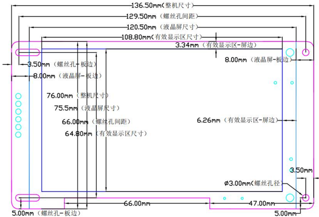
AMZ050 正面图
