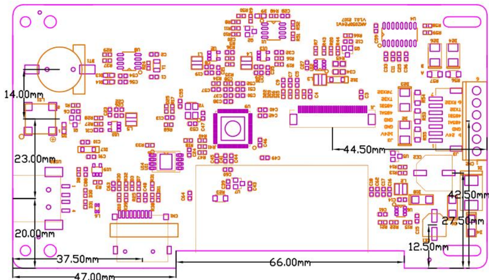
AMZ050 反面图
